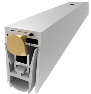
DS-290SF41RQ Square push button in brass Pulsante di spinta quadro in ottone
