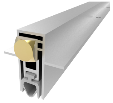
DS-149SF28RQ Square push button in brass Pulsante di spinta quadro in ottone
