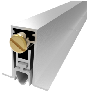
DS-101SF28RT Round push button in brass Pulsante di spinta tondo in ottone
